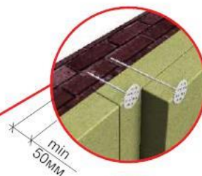
Крепление двух слоев утеплителя
