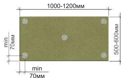
СХЕМА КРЕПЛЕНИЯ УТЕПЛИТЕЛЯ
