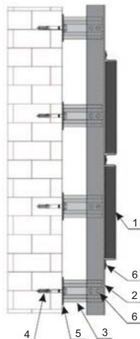
Вид сбоку.
