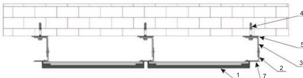
Вид сверху.
